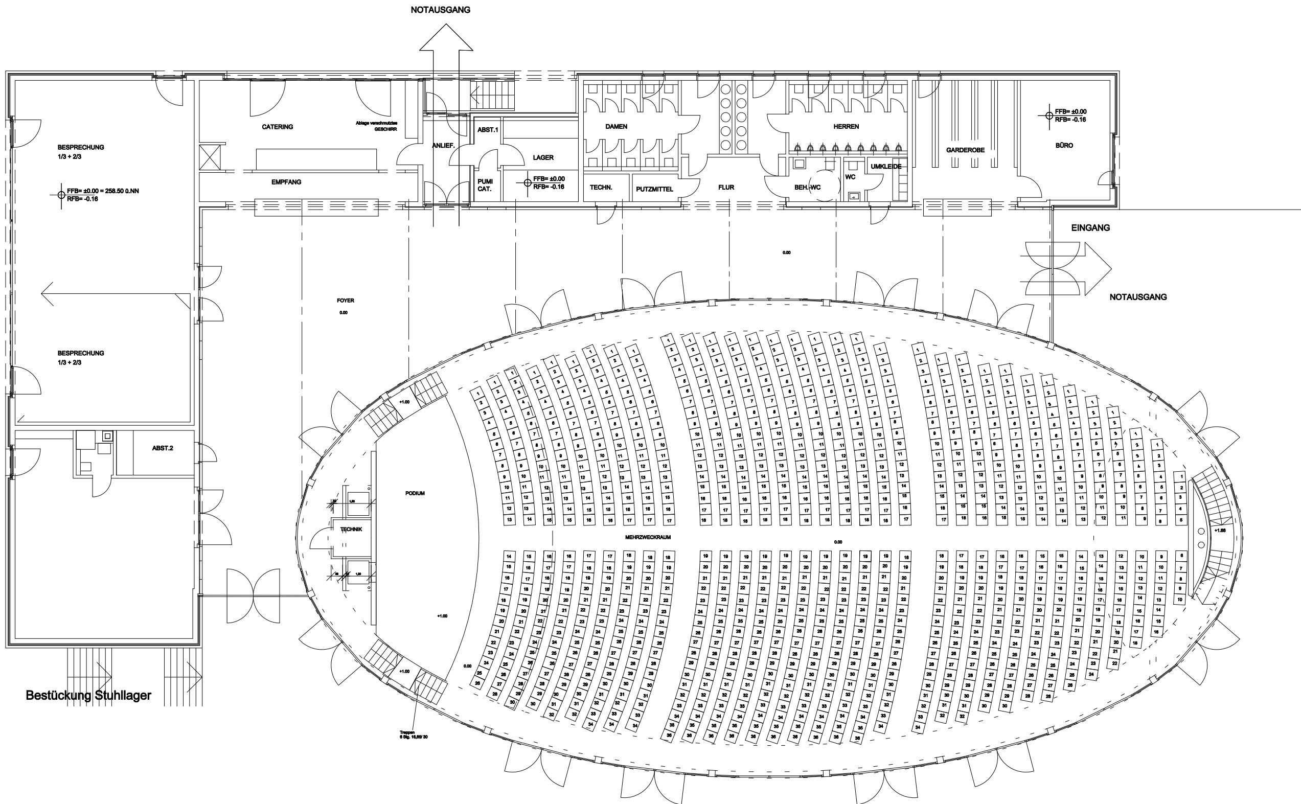
Grundriß Erdgeschoß Reihenbestuhlung mit 1004 Sitzplätzen
